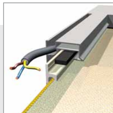
DETAIL GELEIDER + KABEL
